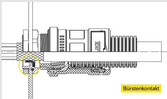
FIPSHIELD® mit EMV Bürste
