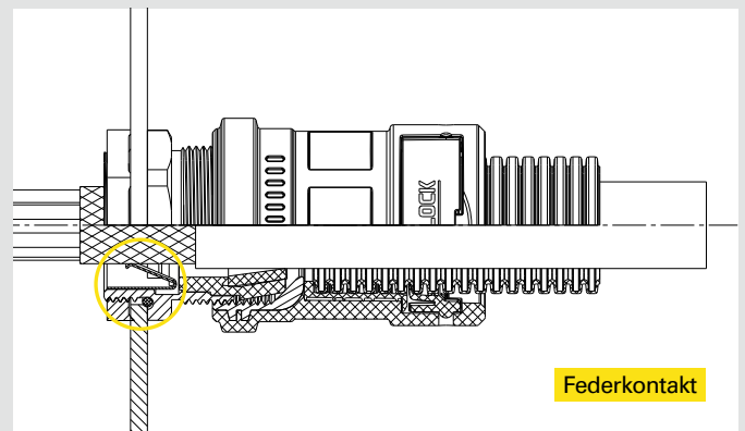
FIPSHIELD® mit EMV Feder
