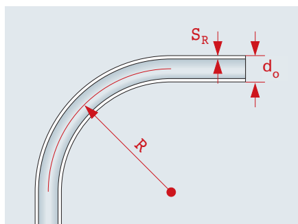
alpex bend radii
